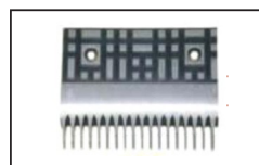
OTAC034 ID:OE-5F 453Y9 Comb AL L127mm W108mm Hole Space 101mm 15T
