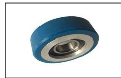
OTRL011 HD Step Roller W AL Hub OD80mm W25mm 6205RZ
