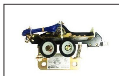
HTLP006 ID:DK-RN4L-A Door Lock
